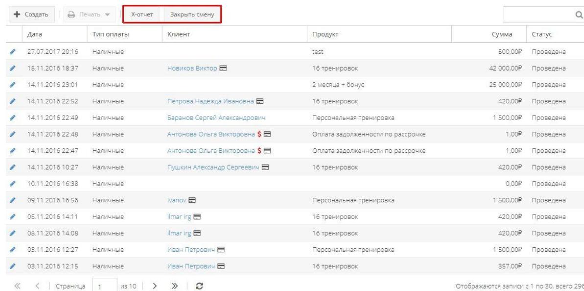
Рис. 7. Печать отчетов
