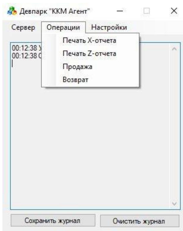
Рис. 4. Меню операций
